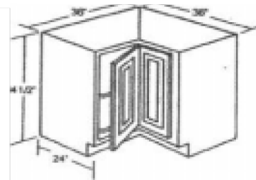
23DCB3612L 36 x 34
